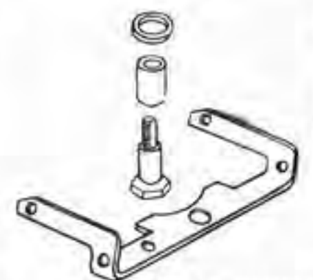
SFN 1158 Biellismo completo destro e sinistro con supporto e viti
