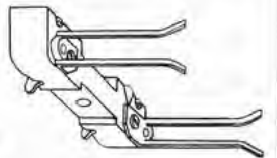
SFN 1039 - Gruppo cilindri con guida per slitta
