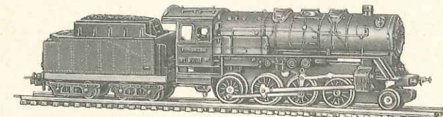
9021 - Locomotiva 5 assi - 9/12 Volts - più tender 4 assi - L. 2.000.
