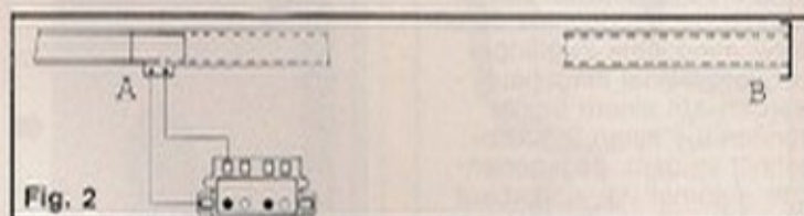
Fig. 2 Schaltplan für Abstellgleis: auf dem zwischen A und B liegenden Abstellgleis fehlt die Stromzufuhr, bis am Stellpult der Druckknopf gedrückt wird. Sonstige würde eine Lokomotive auf dem Abstellgleis stehen bleiben.
